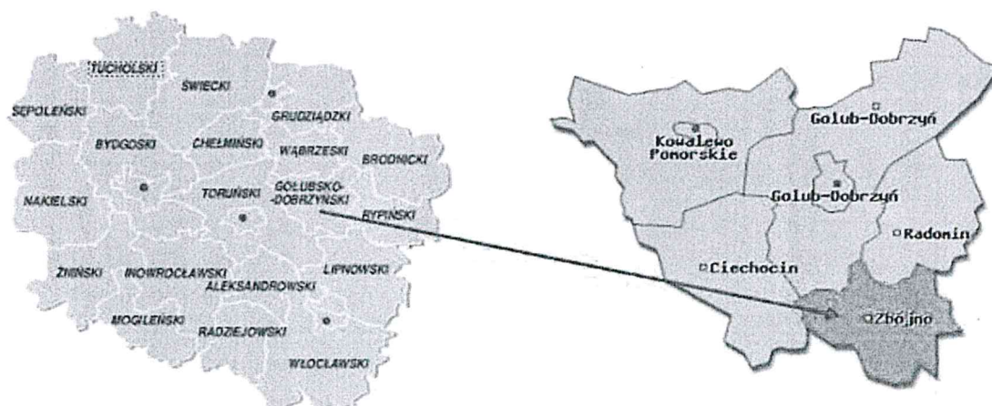
Rysunek 1. Położenie Gminy Zbójno na tle powiatu i województwa
