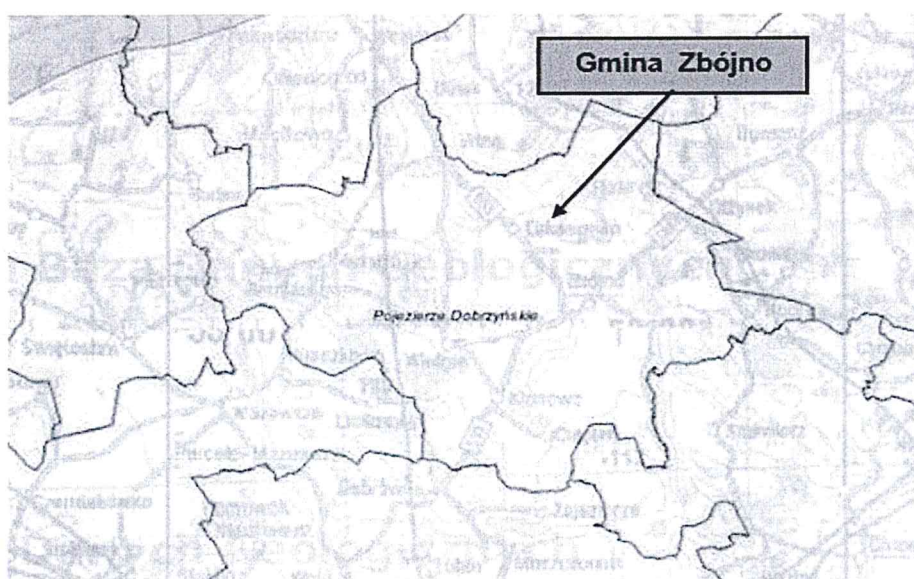
Rysunek 2. Położenie fizyczno-geograficzne Gminy Zbójno
