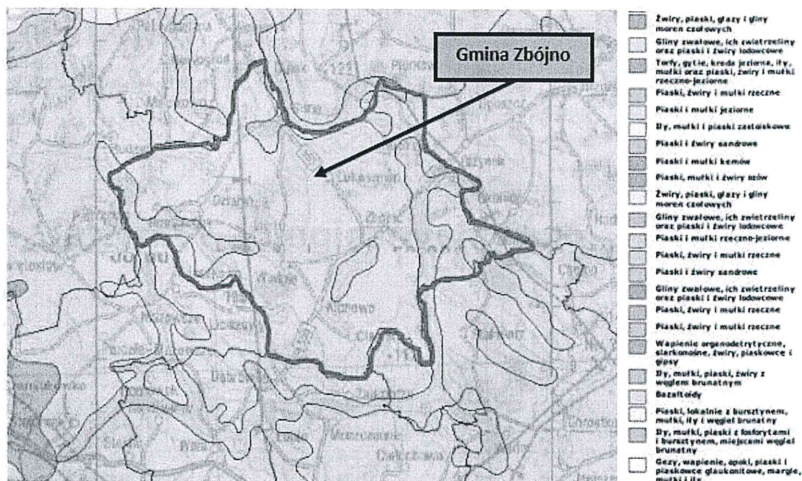
Rysunek 6. Położenie geologiczne Gminy Zbójno
