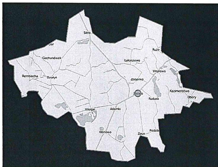
Rysunek 3. Struktura gruntów na terenie Gminy Zbójno
