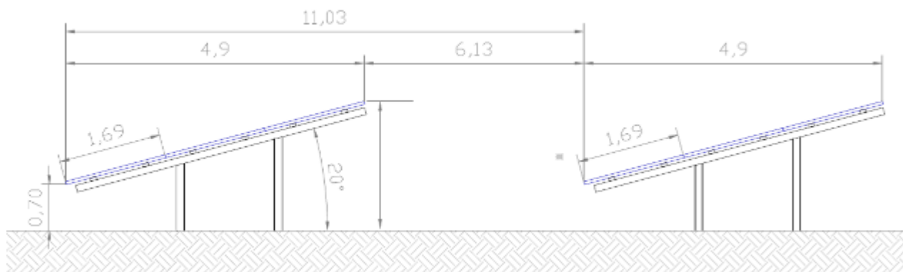
Rysunek 4. Rzut na przykładową konstrukcję stołów z panelami fotowoltaicznymi (rozwiązanie typowe, najczęściej stosowane).
