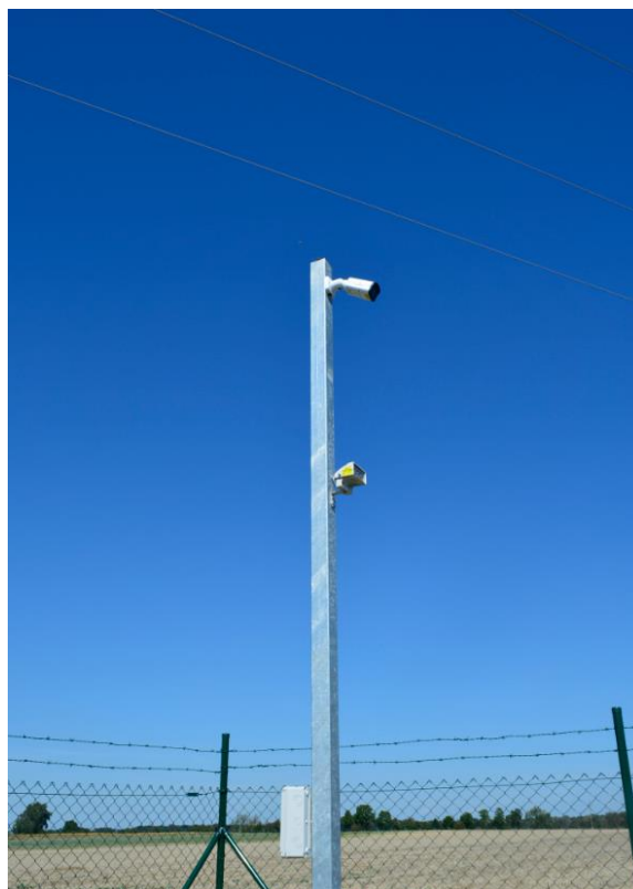
Fot. 3. Widok na zastosowany przykładowy system monitoringu na terenie farmy, farma w miejscowości Olszanka (woj. opolskie) foto: Paweł Kręciproch
